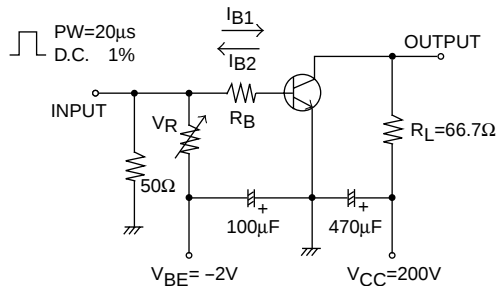
スイッチングタイム測定回路図
