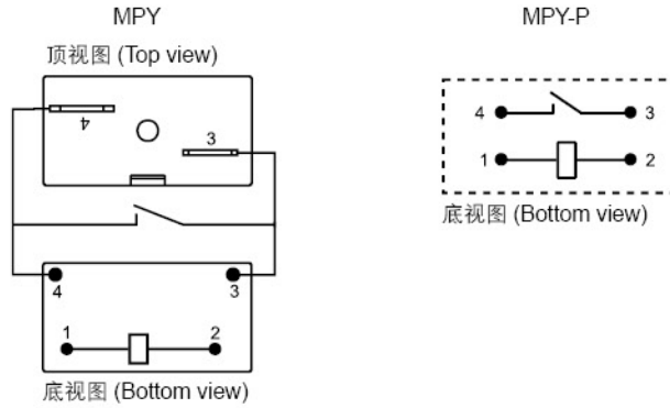
接线图 Wiring Diagram (底视图 Bottom view)
