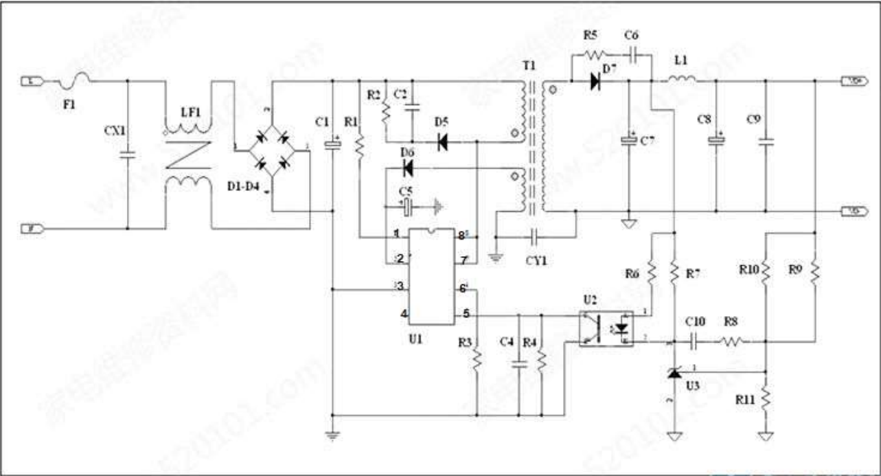
典型应用线路图
