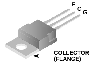
JEDEC TO-220AB
