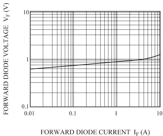
Fig 8. V_F - I_F
