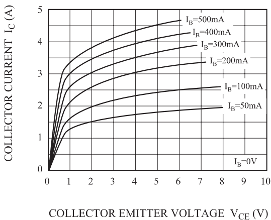
Fig 5. I_C - V_{CE}
