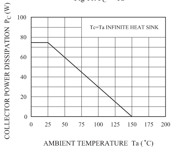
Fig 10. P_C - T_a
