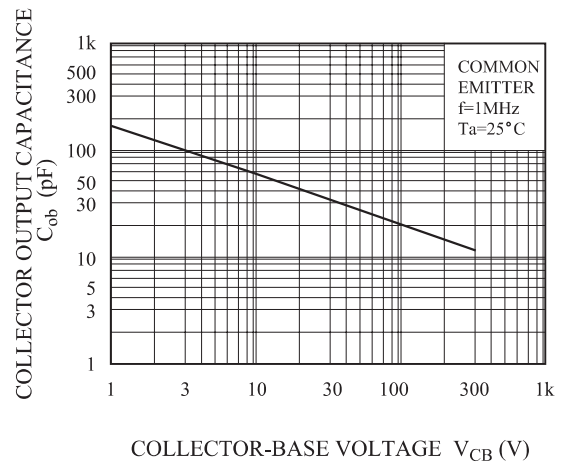
Fig 4. C_{ob} - V_{CB}
