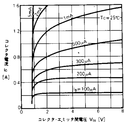
出力特性
