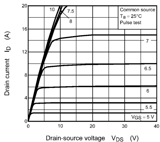
Fig. 8.2 I_D - V_{DS}
