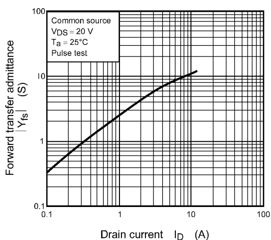
Fig. 8.5 |Y_{fs}| - I_D
