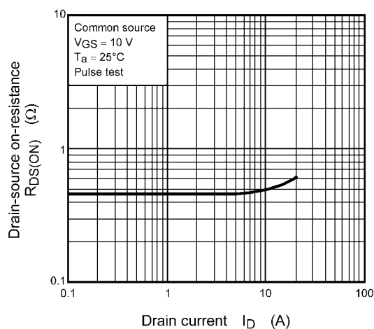
Fig. 8.6 R_{DS(ON)} - I_D
