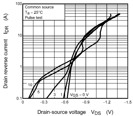
Fig. 8.8 I_{DR} - V_{DS}
