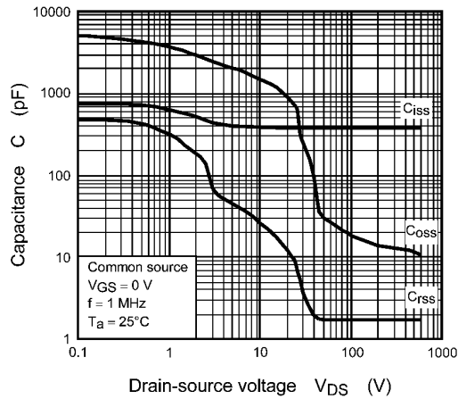
Fig. 8.9 C - V_{DS}
